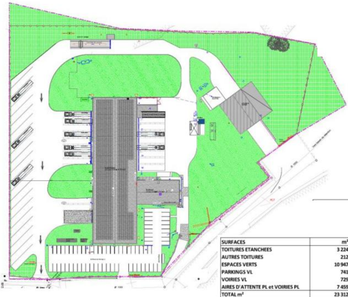
Plan masse
